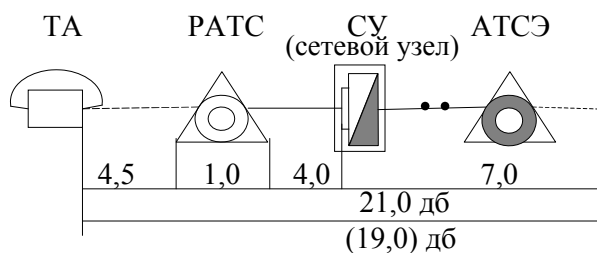
Соединение в пределах районированной сети без узлообразования
