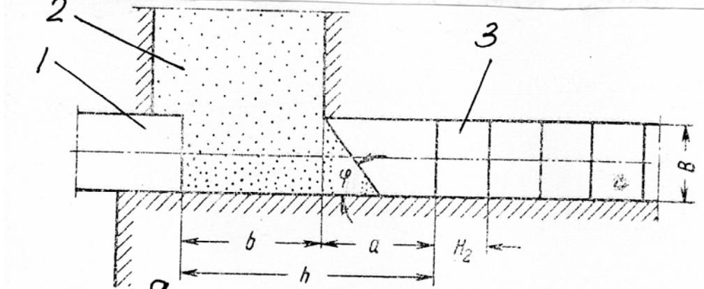
Рис. 4.2. Схема загрузки торфа в матричный канал штемпельного пресса
