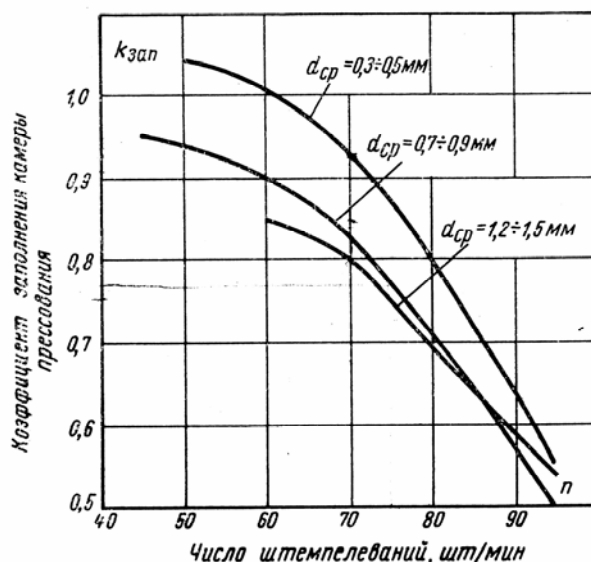
Рис. 4.3. Влияние скорости прессования n (штемпелеваний в 1 мин) на коэффициент заполнения камеры прессования k_{зап} для высушенного торфа с различным средним диаметром частиц d_{ср}
