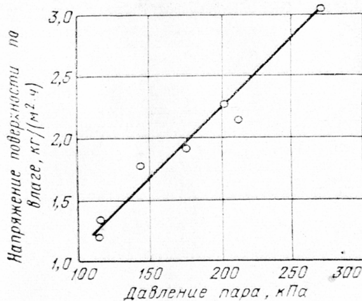
Рис. 4.1. Зависимость между напряжением поверхности нагрева паровой трубчатой сушилки и давлением пара
