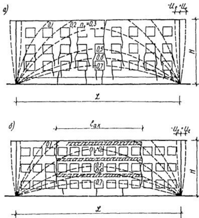
Рис. 16. Напряженное состояние ( n_i ), деформации ( U_t ) и развитие трещин в стенах каменных зданий при температурно-влажностных воздействиях
