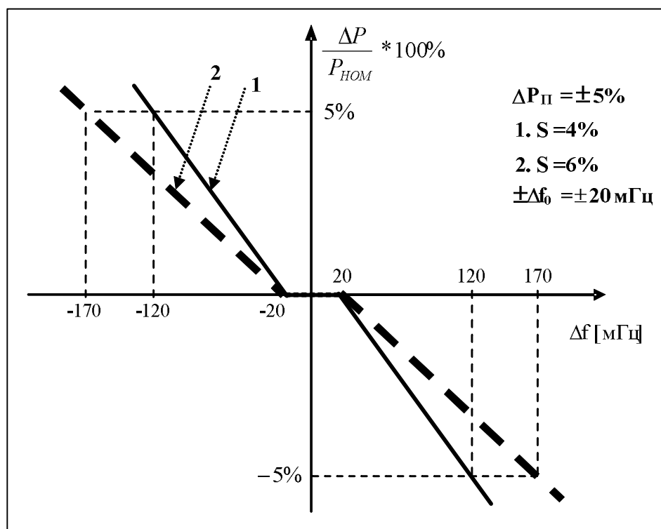
Рис. 4.3. Статическая характеристика первичного регулирования для разных величин статизма.
