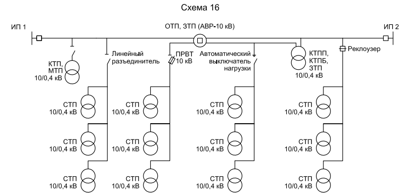
Рисунок 14 – Схема сети с переносом источников трансформации (СТП 10/0,4 кВ) к потребителю в сельских населенных пунктах
