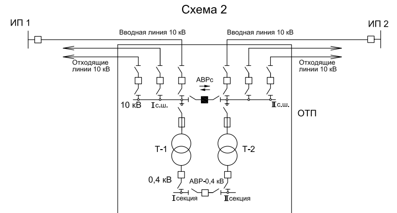
Рисунок 2 – Схема присоединения ТП 10/0,4 кВ, питающей потребителей категории 1
