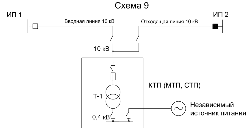
Рисунок 9 – Схема присоединения ТП 10/0,4 кВ, питающей потребителей категории 2
