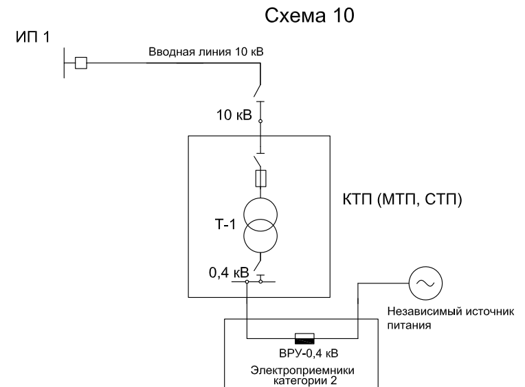
Рисунок 10 – Схема присоединения ТП 10/0,4 кВ, питающей потребителей категории 2
