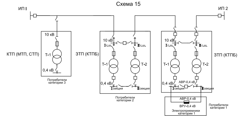
Рисунок 13 – Схема сети 10 кВ с подключением потребителей категорий 1, 2 и 3
