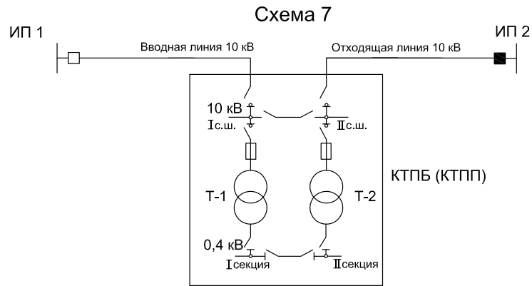
Рисунок 7 – Схема присоединения ТП 10/0,4 кВ, питающей потребителей категории 2
